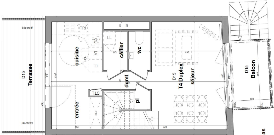
Plan D15 bas R+1
