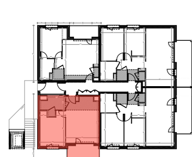
Niveau R+2
