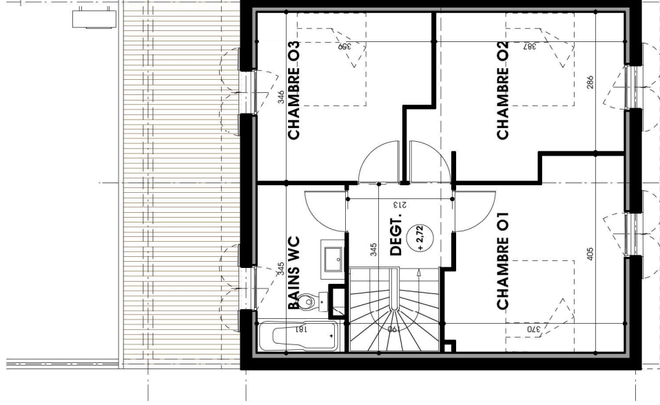
ÉTAGE
