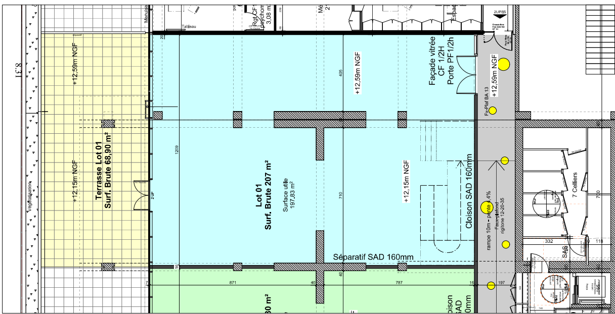
Plan LOT 01 - 1/100 Surface Brute : 207,00 m 2 Surface Utile : 197,83 m 2 Terrasse : Surface Brute : 68,90 m 2
