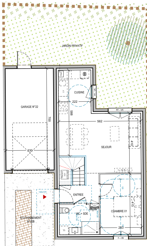
REZ-DE-CHAUSSEE
