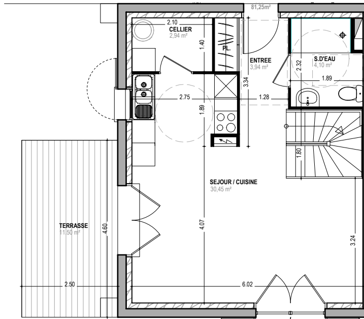
PLAN - RdC
