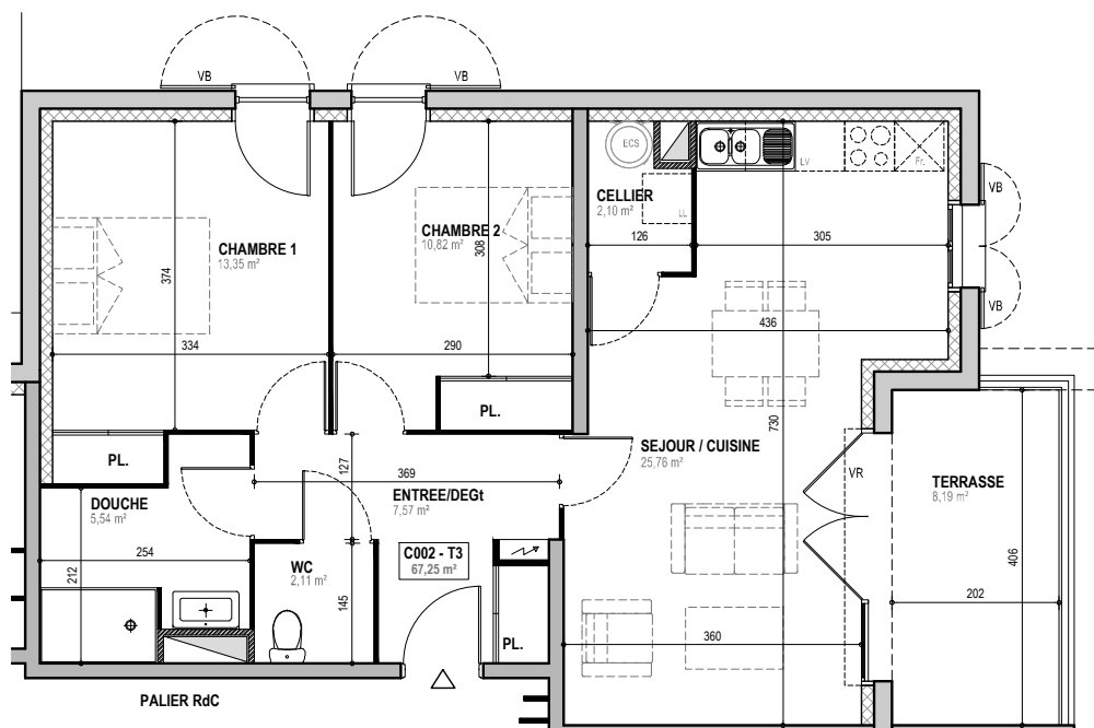
PLAN - RdC
