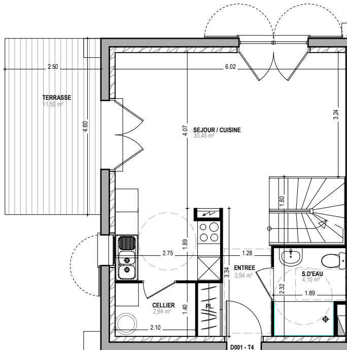
PLAN - RdC
