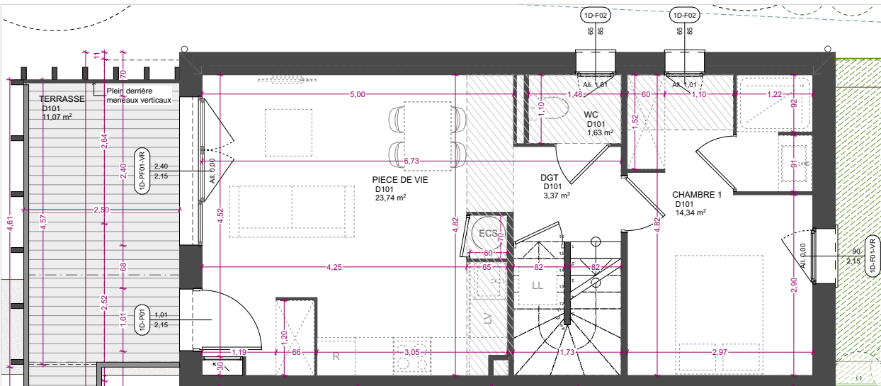
niveau R+1
