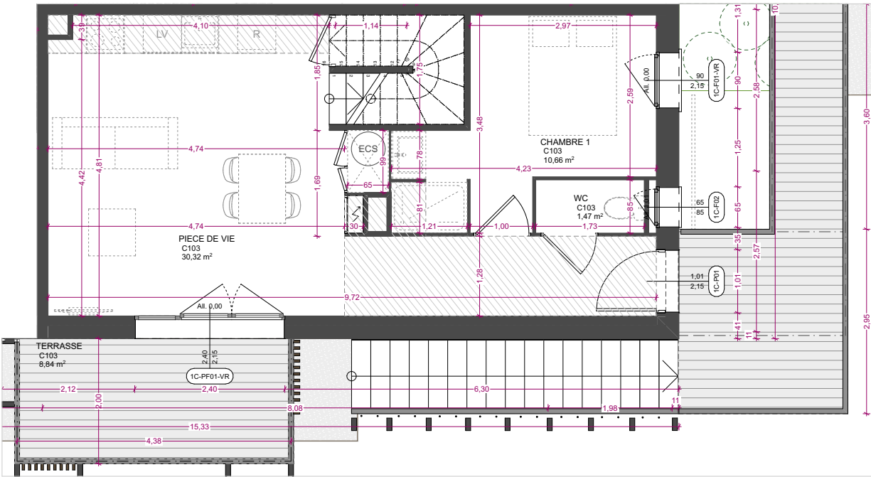
niveau R+1
