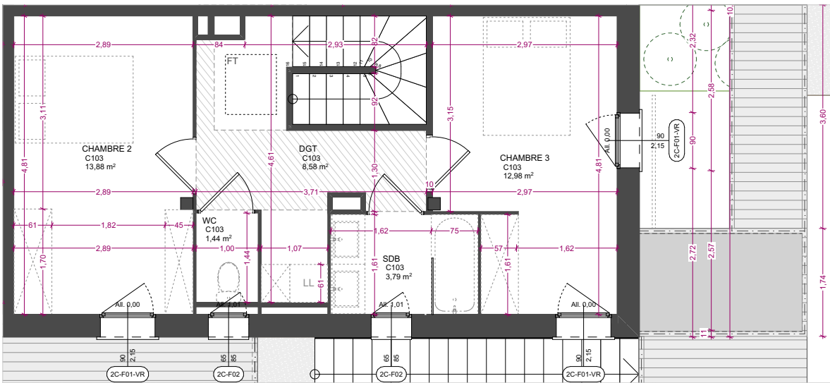
niveau R+2
