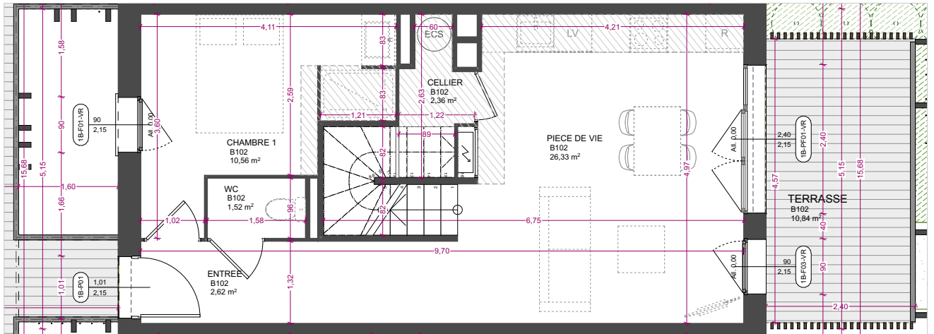
niveau R+1
