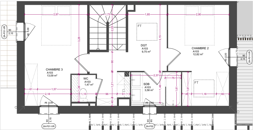
niveau R+2
