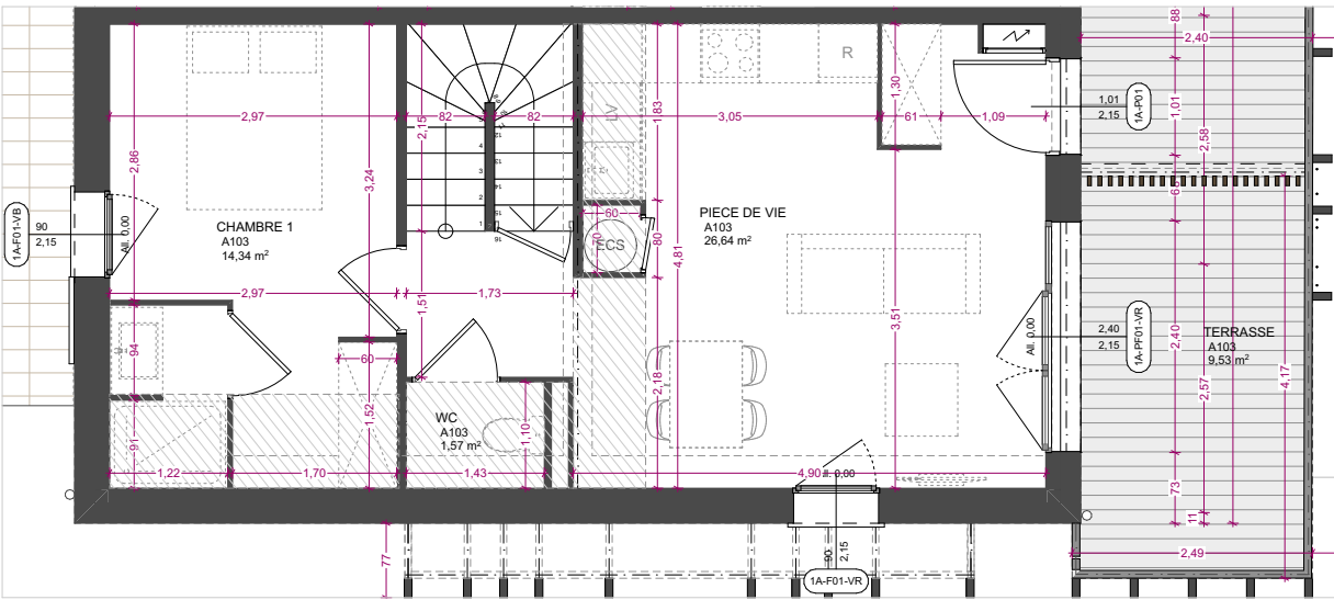
niveau R+1
