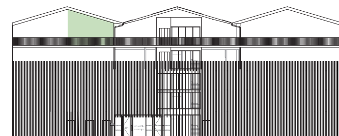
Façade NORD
